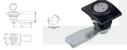
Silindir Yaylı Pano Kilidi / Plastik Kare Gövde
