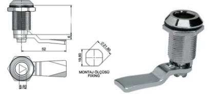
Yaylı Pano Kilidi / 40mm
