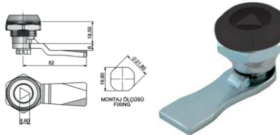
Yaylı Pano Kilidi / Üçgen Statik Boyalı
