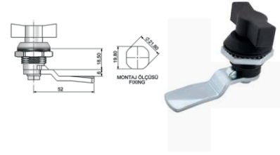
Mini Yaylı Pano Kiliti / Plastik Kelebek
