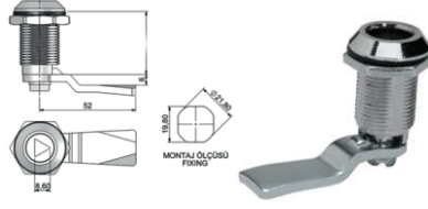
Yaylı Pano Kilidi / 35mm
