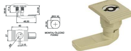
Yaylı Pano Kilidi / Dörtgen RAL-7032
