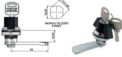
Silindir Yaylı Pano Kilidi / Kelebek
