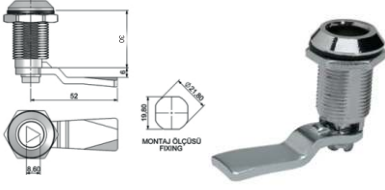
Yaylı Pano Kilidi / 30mm
