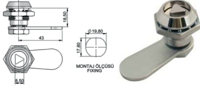
Bilyalı Pano Kilidi / Üçgen
