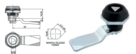
Plastik Yaylı Pano Kilidi / Üçgen Göbekli
