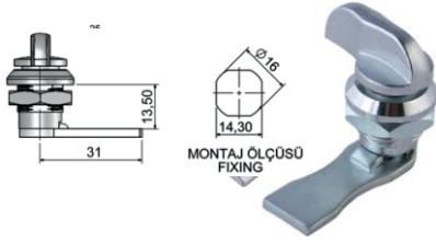
Mini Yaylı Pano Kiliti
