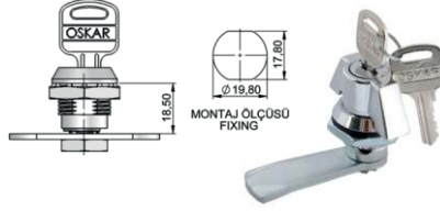
Silindir Yaylı Pano Kilidi / Kelebek
