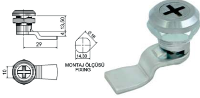
Mini Yaylı Pano Kilidi / Tornavida Başlı
