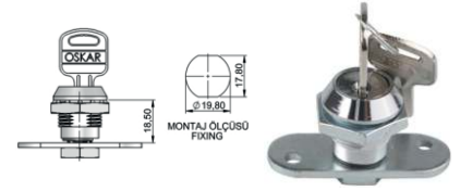
Mandallı Kilit Eğri Dilli / İspanyolek
