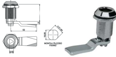
Yaylı Pano Kilidi / 60mm
