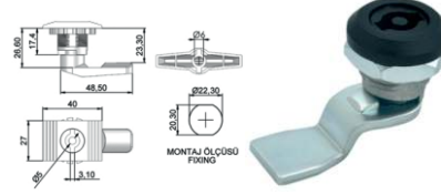
Mini Yaylı Pano Kilidi / Tornavida Başlı Statik Boyalı
