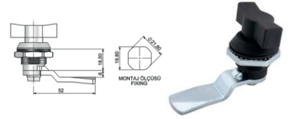
Yaylı Pano Kilidi / Plastik Kelebek
