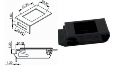
Sürgü Kilit / 1.2 mm
