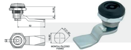
Yaylı Pano Kilidi / Plastik DB
