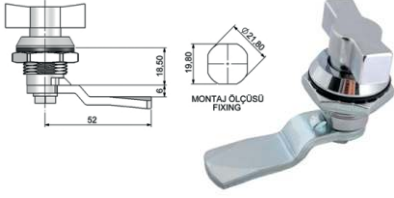
Yaylı Pano Kilidi
