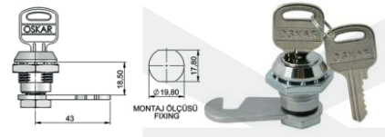
Mandallı Kilit / Şifreli ve Sekmalı
