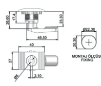
Yaylı Pano Kilidi / Dörtgen
