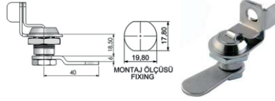
Mandallı Kilit Eğri Dilli / Asthma Hamilli
