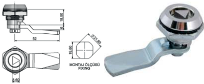
Yaylı Pano Kilidi / Üçgen
