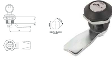
Silindir Yaylı Pano Kilidi / Plastik Gövde
